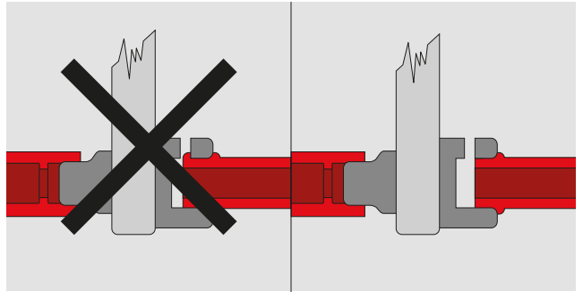
No superar el borde exterior de la boquilla ranurada.
